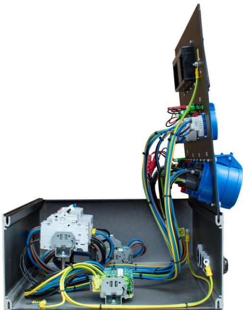
Seitenansicht eines Versatzkastens mit LSS VK-Profil 155
